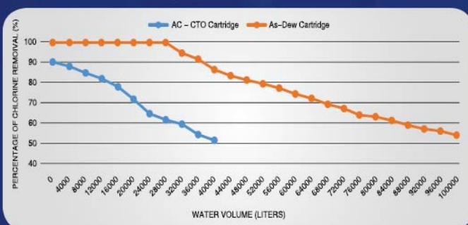
除氯效率曲线图
